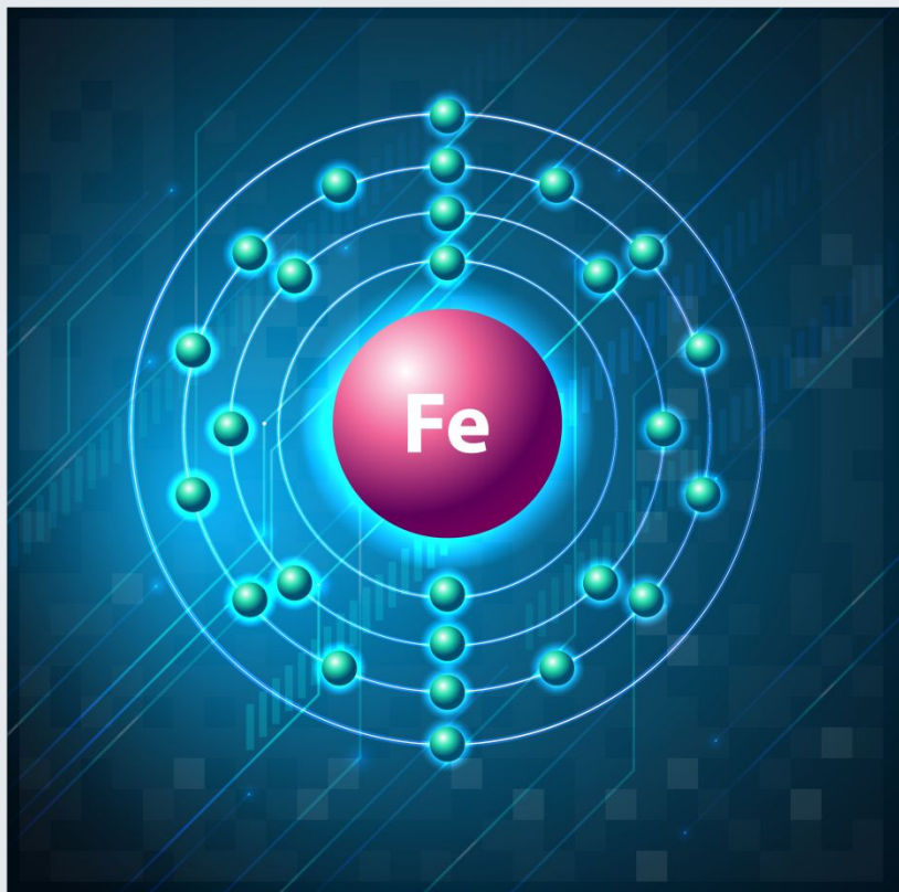
атом железа
