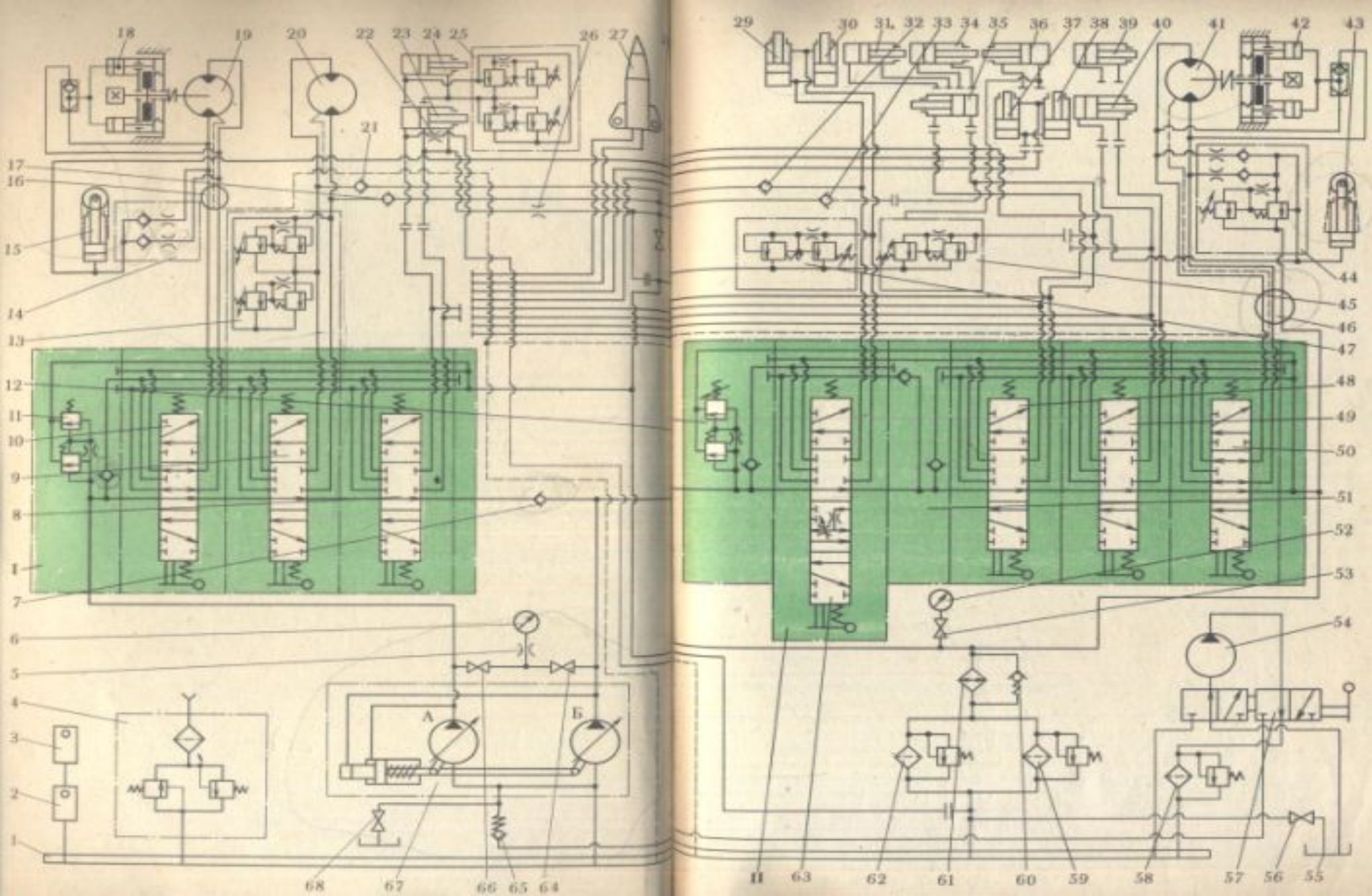
Рис. 5 Гідравлічна схема екскаватору
