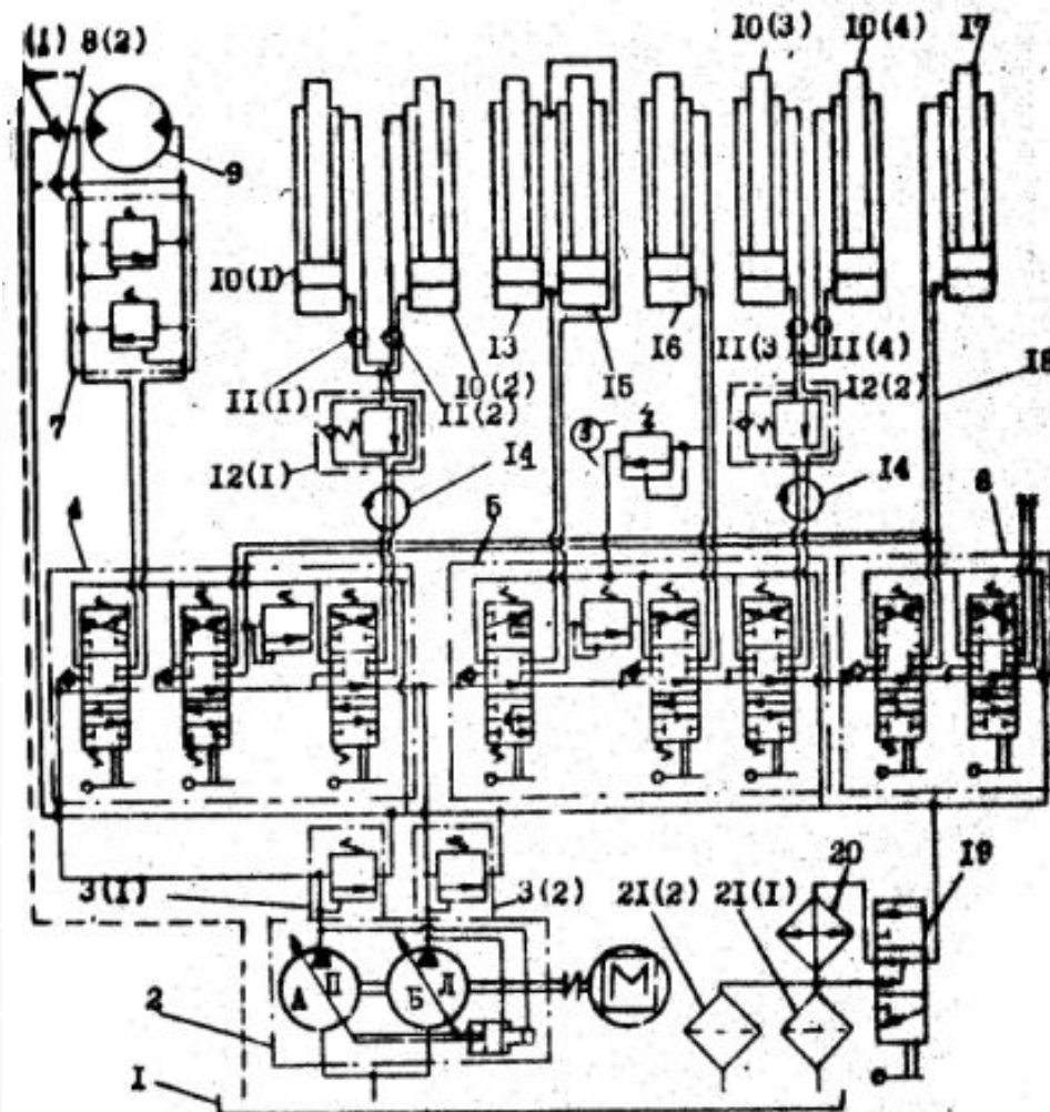
Рис. 12 Схема гідравлічна принципова:
