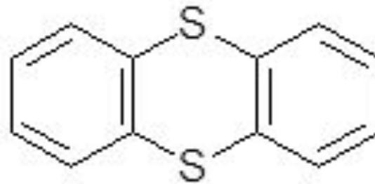
Сернистые красители
