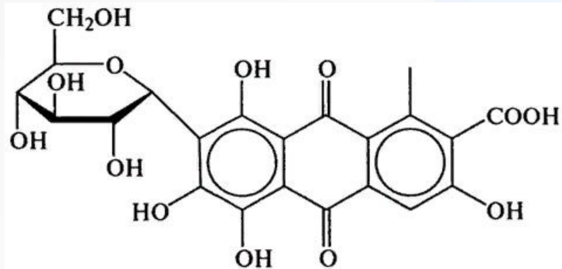
карминовая кислота
