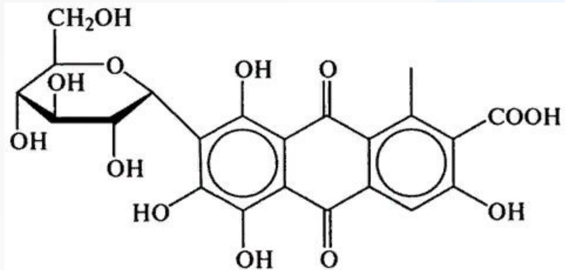
карминовая кислота
