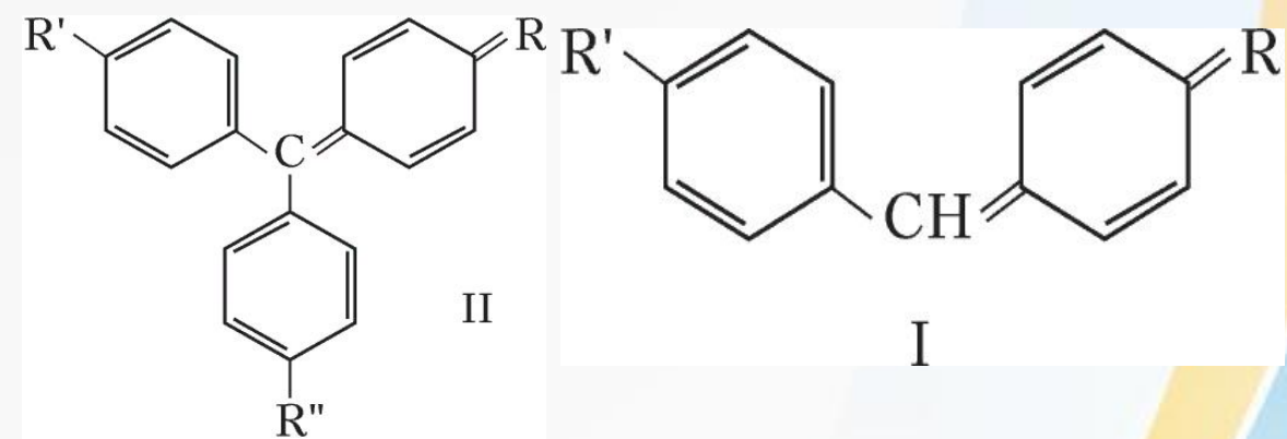
Арилметановые красители
