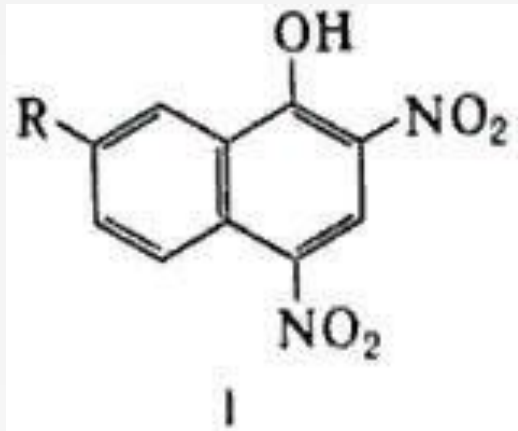
Нитрокрасители
