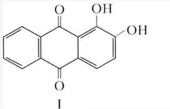
Антрахиноновые красители
