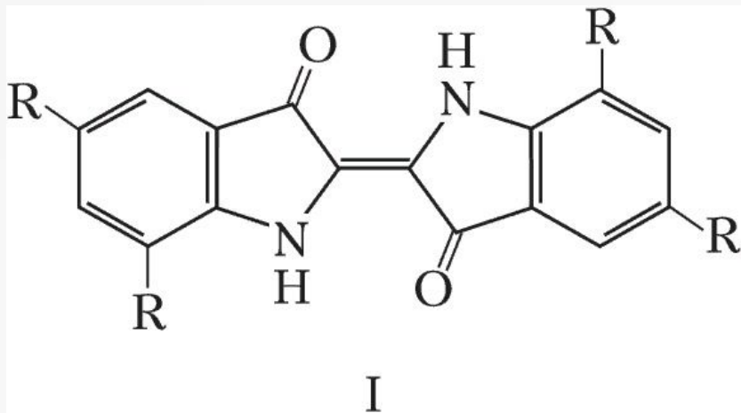
Индигоидные красители
