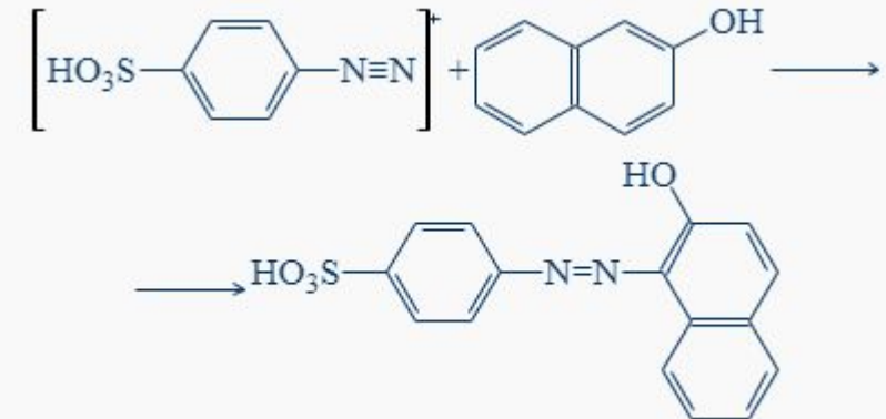
Азокрасители
