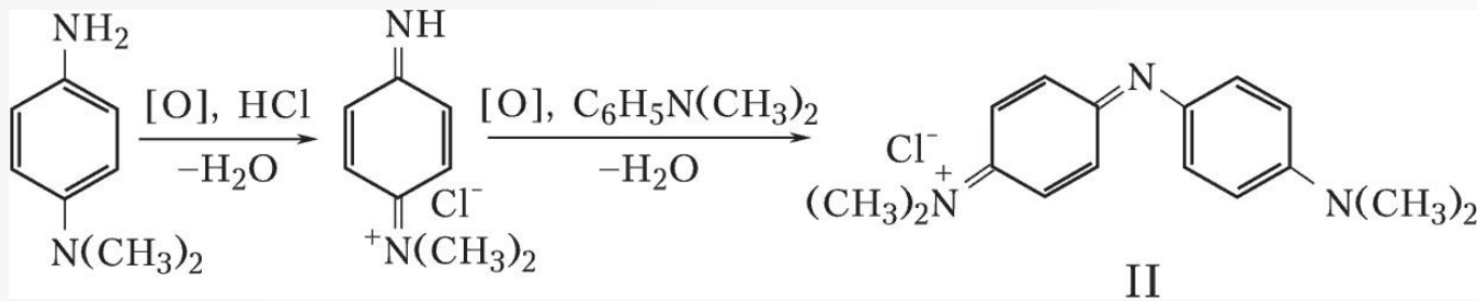
Хинониминовые красители
