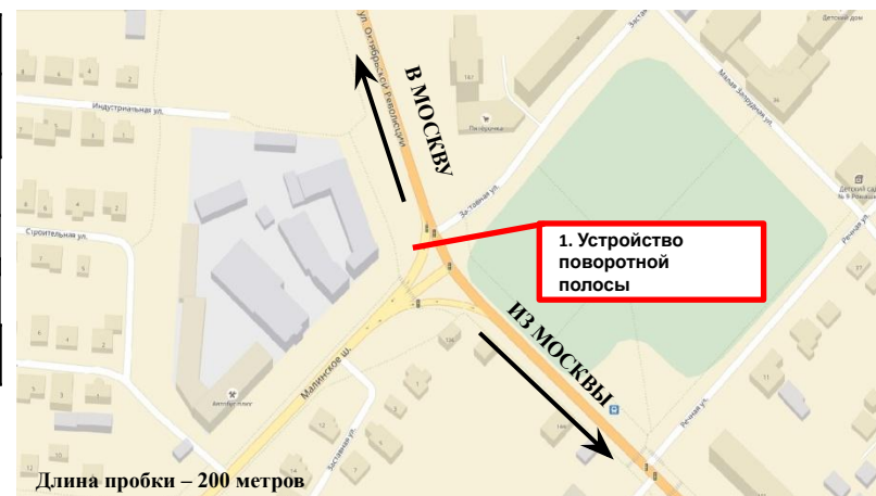
Существующая схема движения
