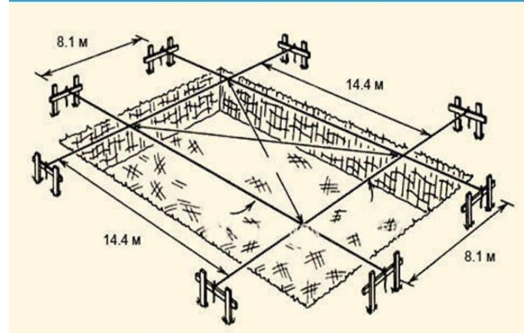
Разметка участка под фундамент
