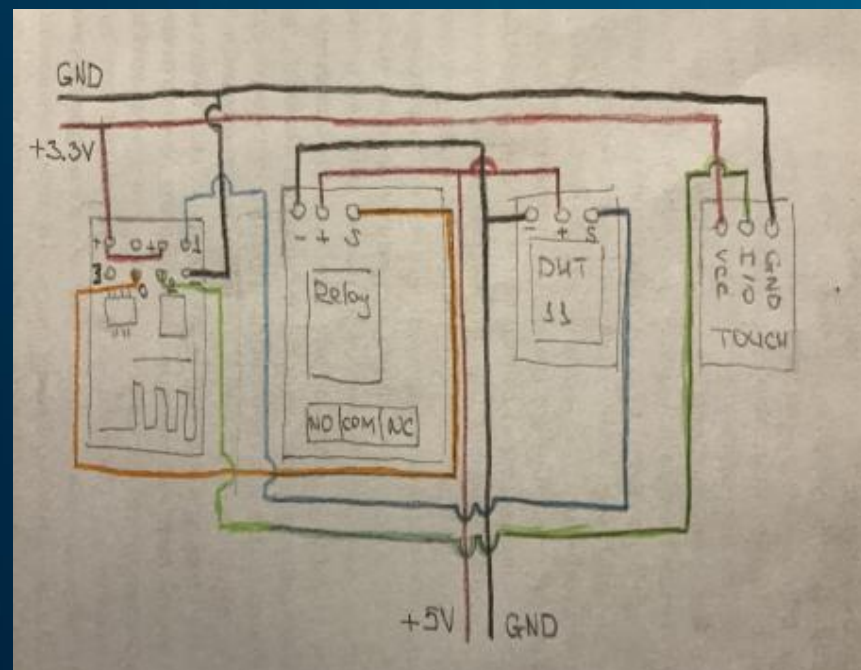
Схема модуля умного дома на базе ESP-01 Электронный выключатель с термометром
