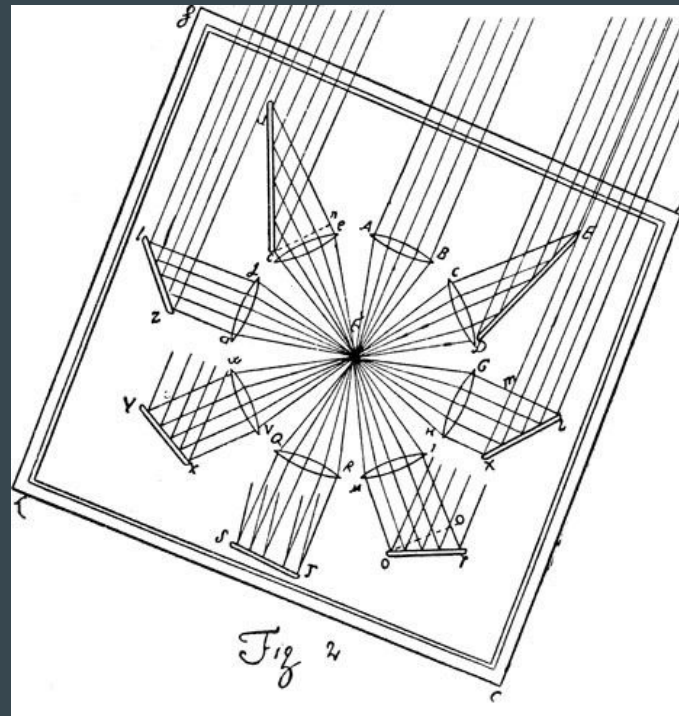
Проект зажигательного катоптрико-диоптрического инструмента
