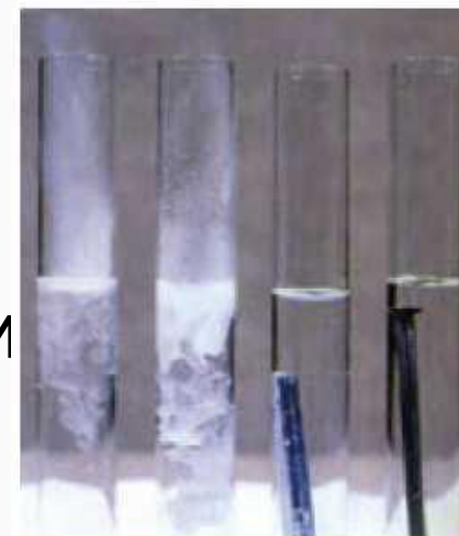
Рис. 36.3. При обычных условиях натрий и кальций активно взаимодействуют с водой с выделением водорода, а цинк и железо не взаимодействуют
