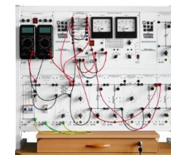
Стенд для подготовки электромонтажников
