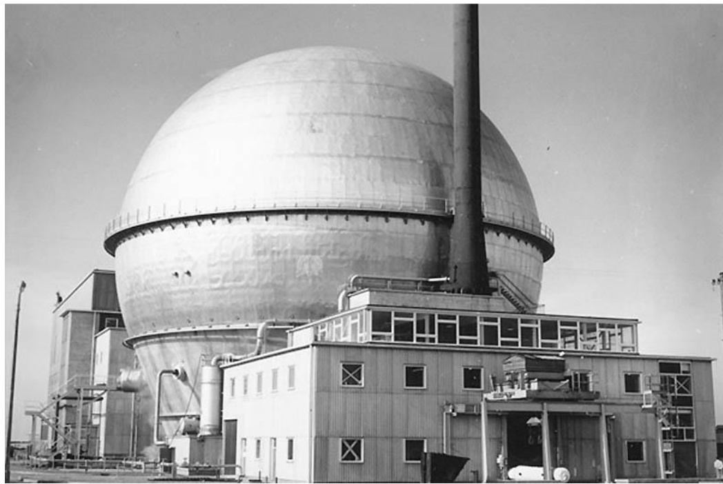
ёмкости для радиоактивных отходов
