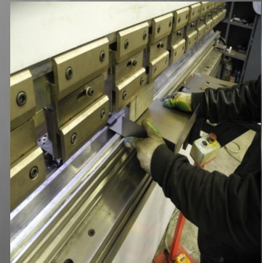
Пресс листогибочный INGRO XS-2060
