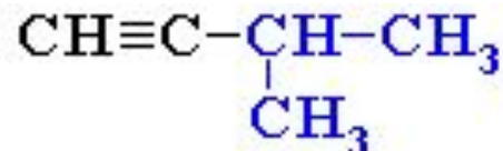
3-метилбутин-1
