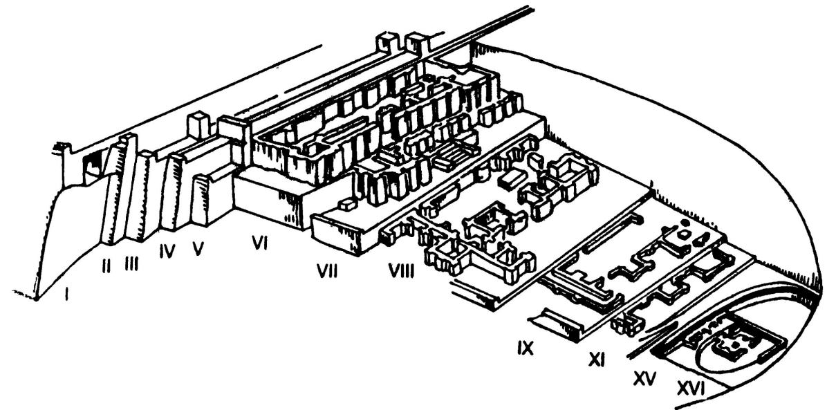
Рис. 6. Схема напластований на храмовом участке Эреду
