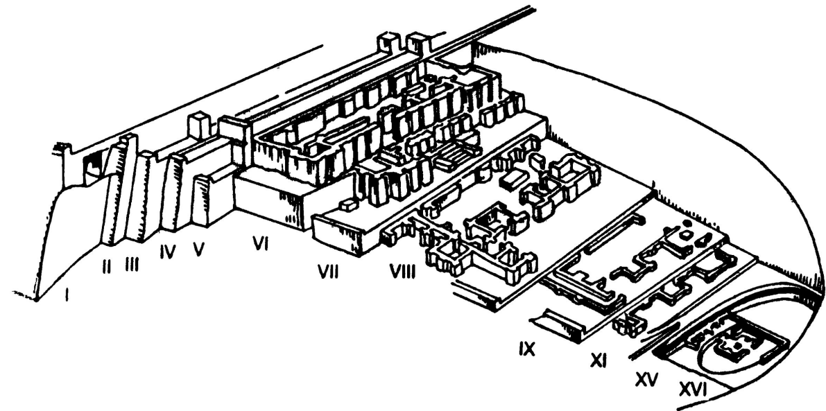
Рис. 6. Схема напластований на храмовом участке Эреду
