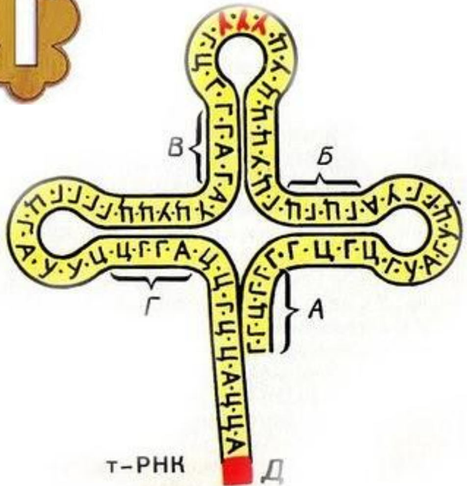
Схема Т-РНК.
