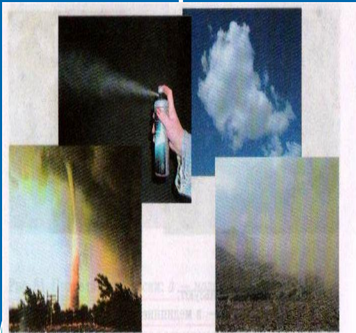
Рис. 85. Аэрозоли
