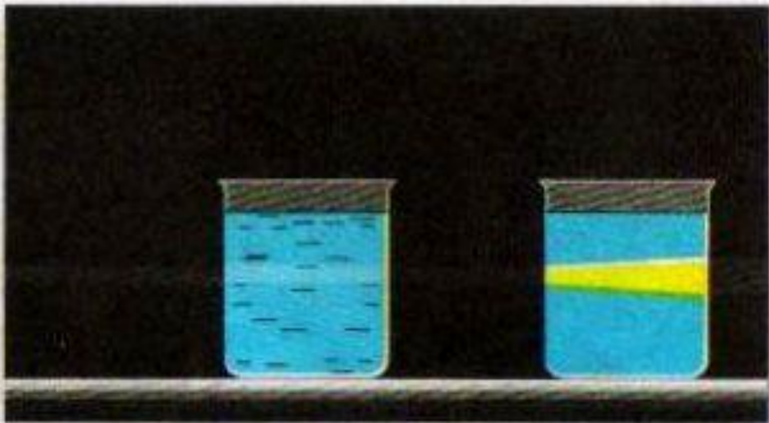
Рис. 88. Эффект Тиндалля
