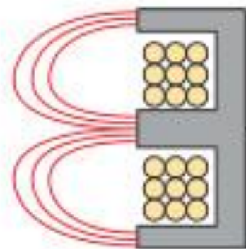
Катушка индуктивности с открытым магнитопроводом
