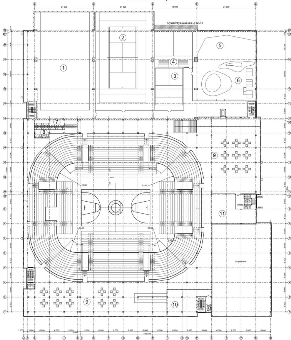
План на отм. +7,600
