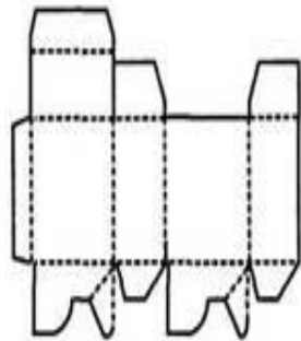
Дно замкового типа
