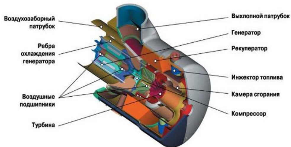
Конструкция микротурбинного двигателя
