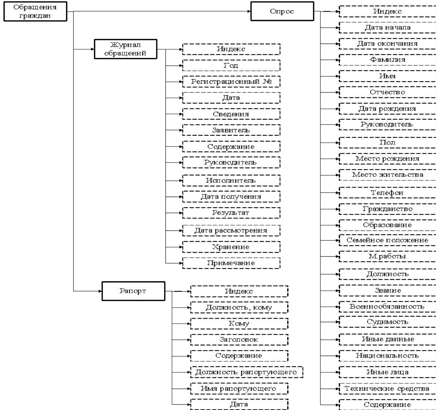
Инфологическая модель
