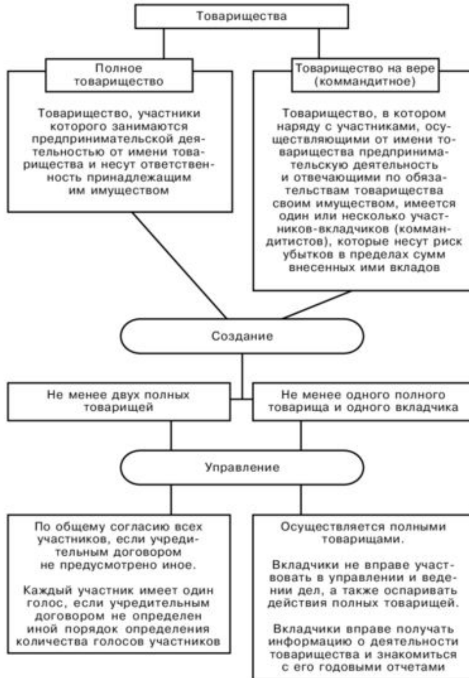
Рис. 3.4. Хозяйственные товарищества
