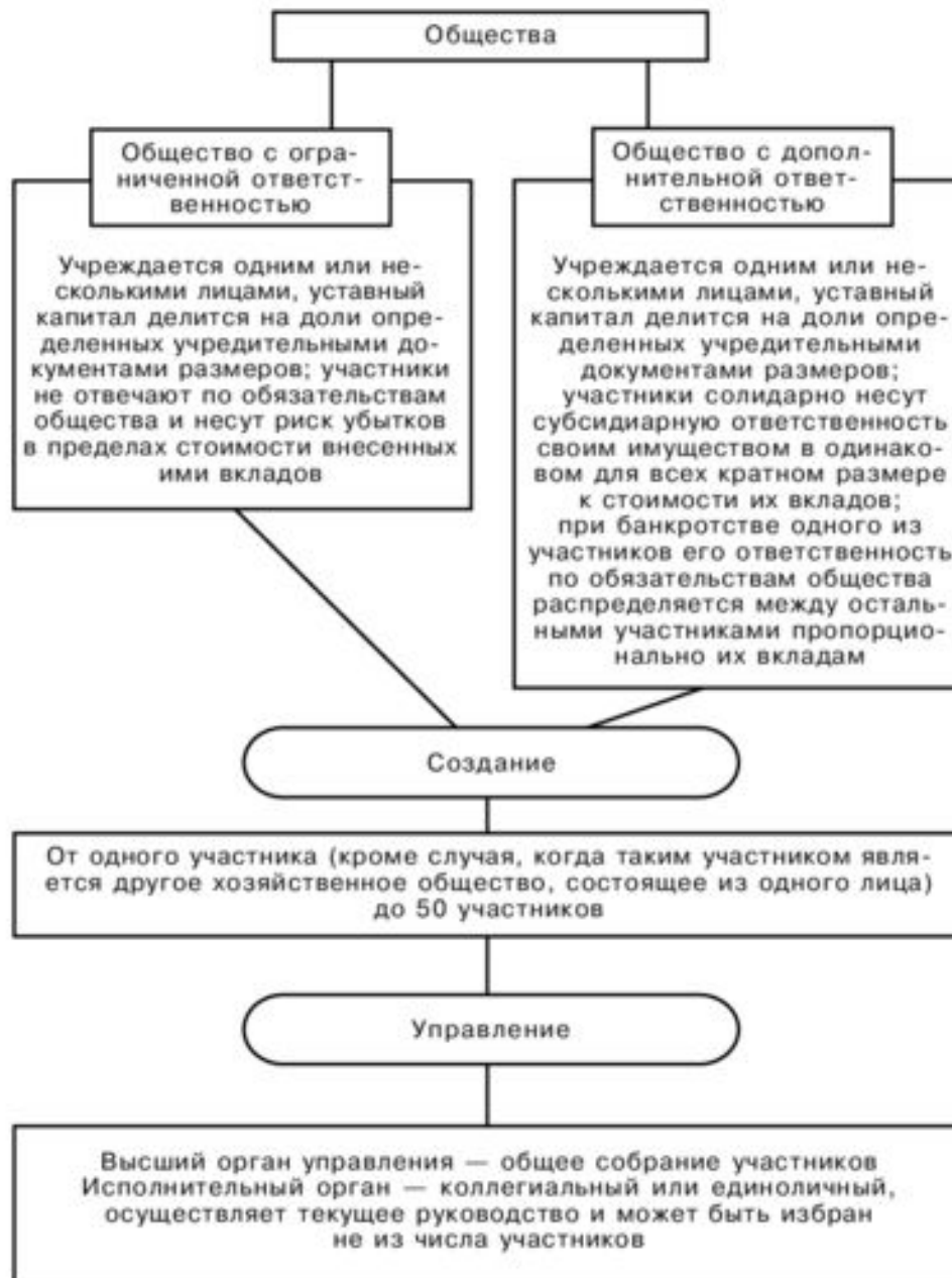
Рис. 3.5. Хозяйственные общества
