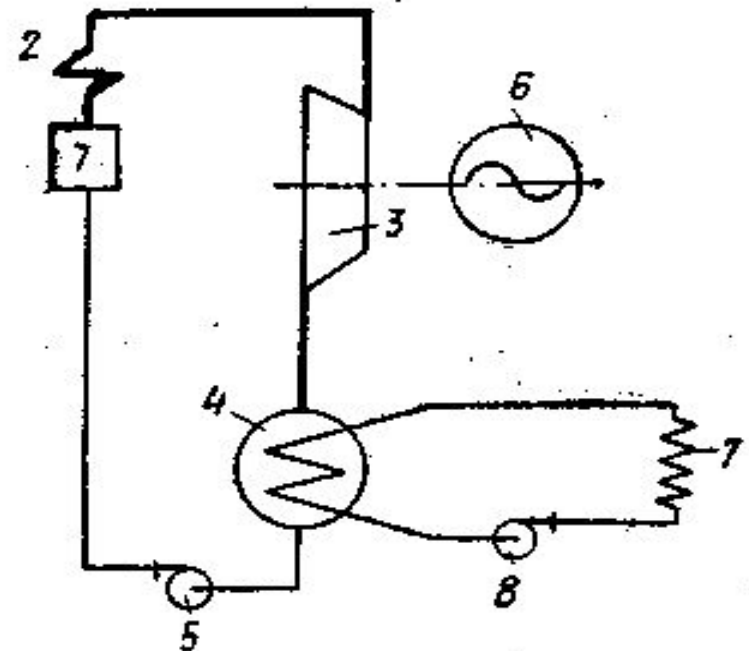
Рис. 10-24. Схема простейшей теплофикационной установки
