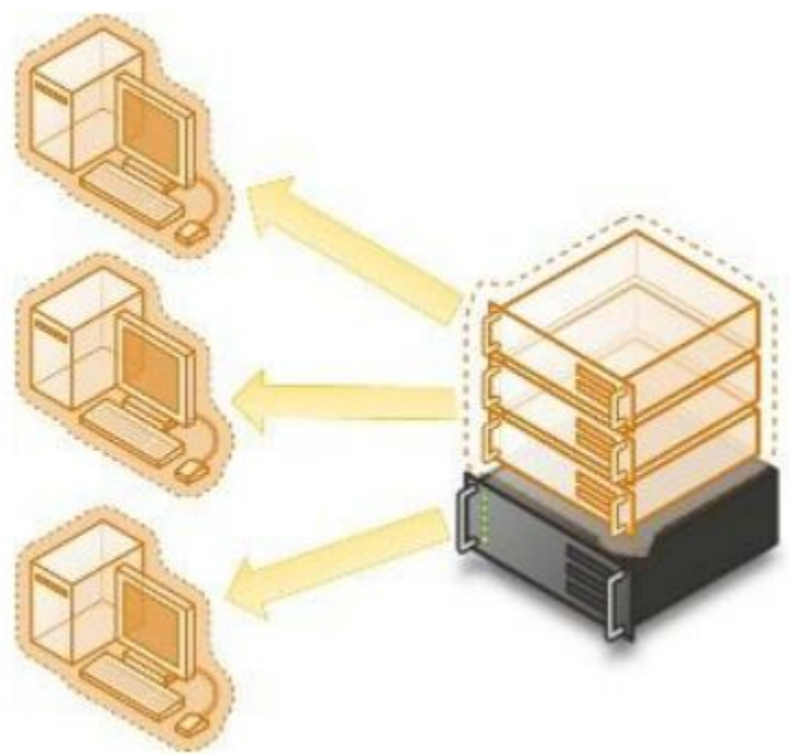
Рисунок 2.8 Виртуализация представлений
