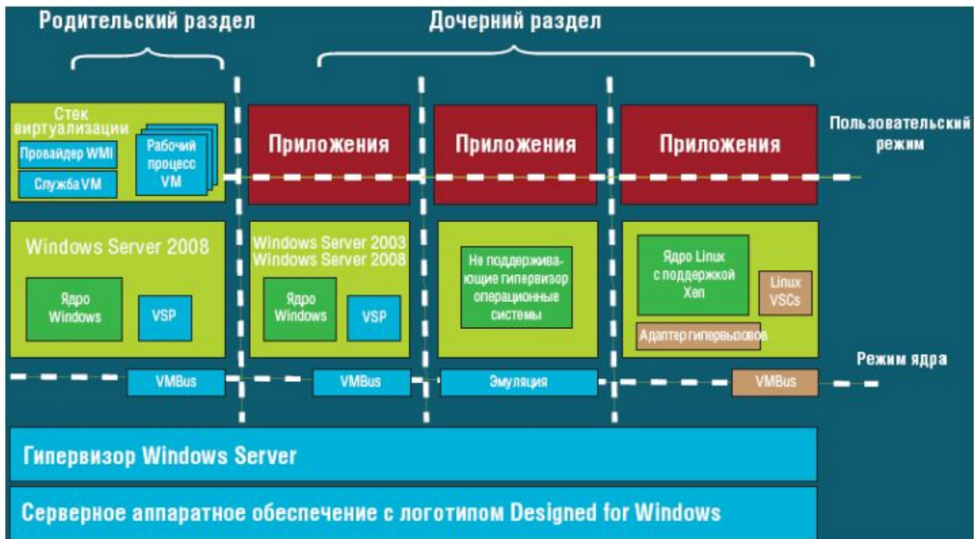
Рисунок 2.15 Архитектура Hyper-v
