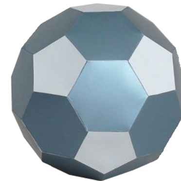
Усечённый икосаэдр
