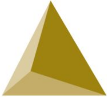
Правильный тетраэдр
