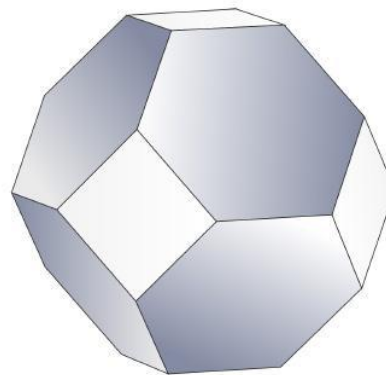
Усечённый октаэдр
