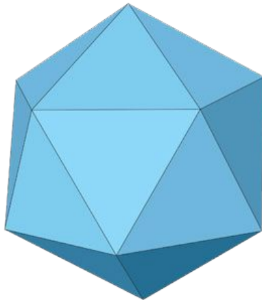
Икосаэдр
