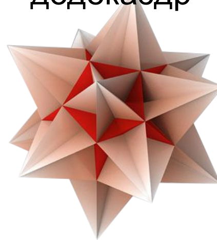
Большой икосаэдр
