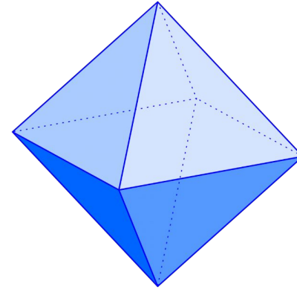
Октаэдр
