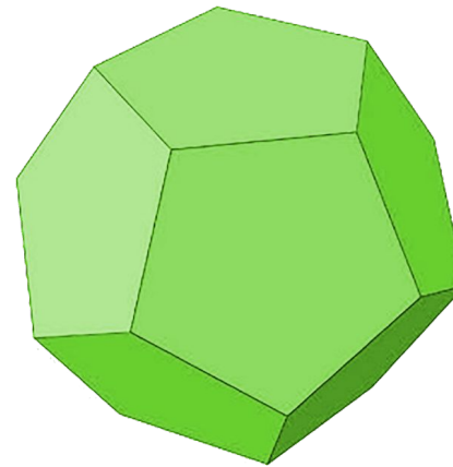
Додекаэдр
