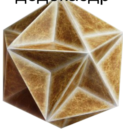
Большой додекаэдр
