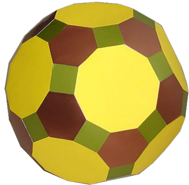
Ромбоусечённый икосододекаэдр
