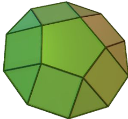
Пятискатный купол
