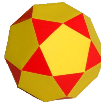
Икосододекаэдр
