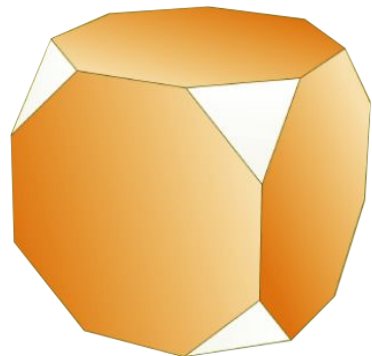
Усечённый гексаэдр
