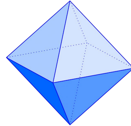
Октаэдр
