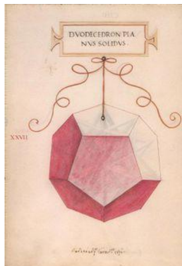
Многогранники на иллюстрациях Леонардо да Винчи
