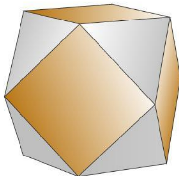
Кубооктаэдр
