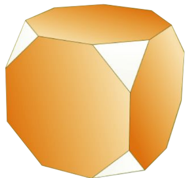
Усечённый гексаэдр
