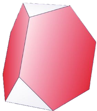
Усечённый тетраэдр
