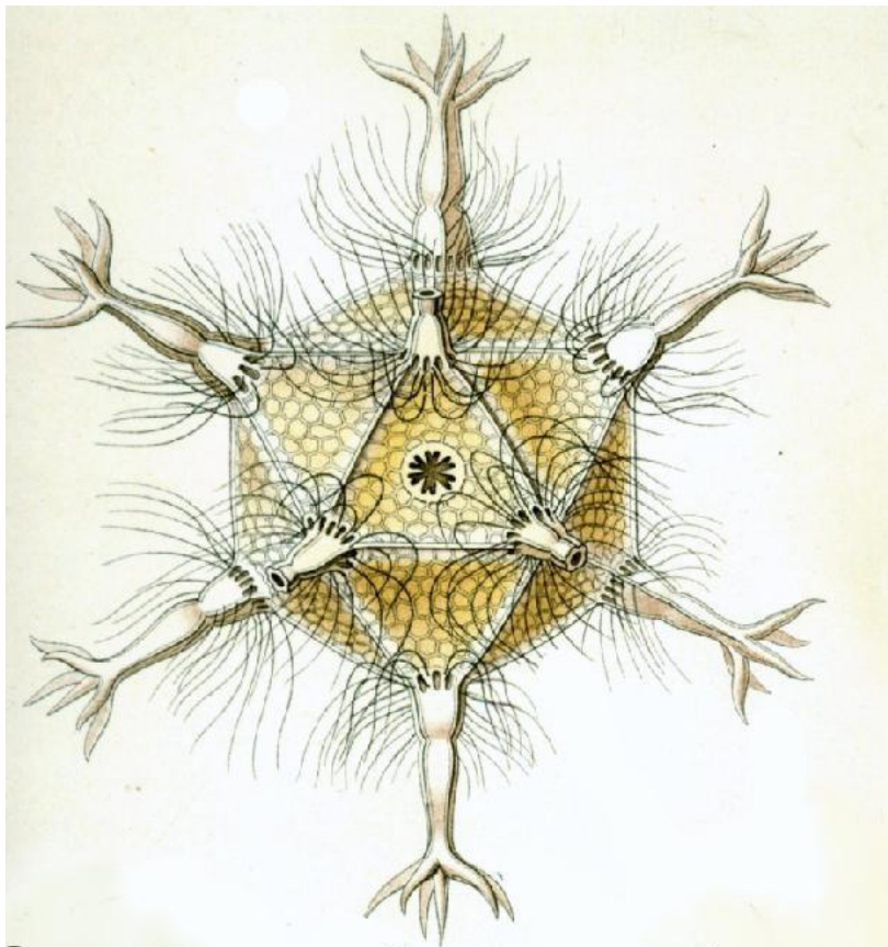
Феодария
