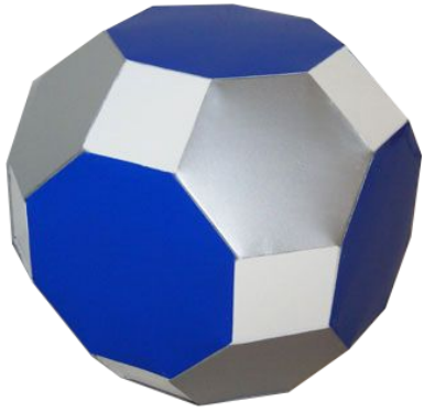
Ромбоусечённый кубооктаэдр
