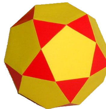
Икосододекаэдр
