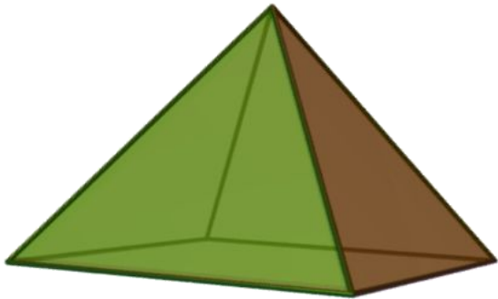
Квадратная пирамида
