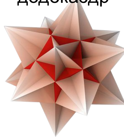
Большой икосаэдр
