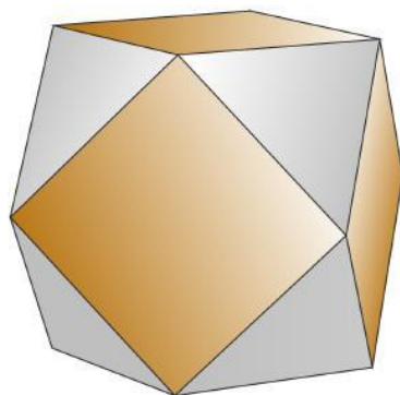
Кубооктаэдр
