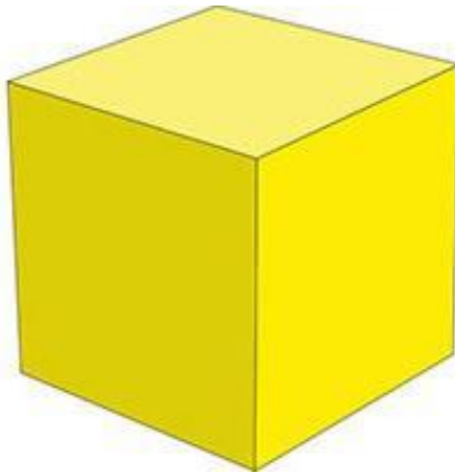
Гексаэдр (куб)
