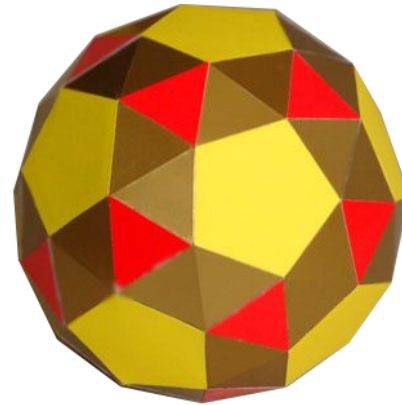
Плосконосый додекаэдр
