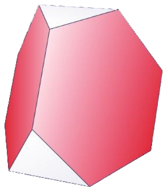
Усечённый тетраэдр
