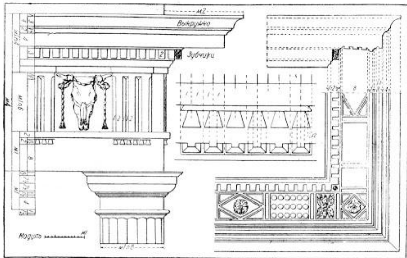
Капитель и антаблемент дорического ордера (зубчатого)
