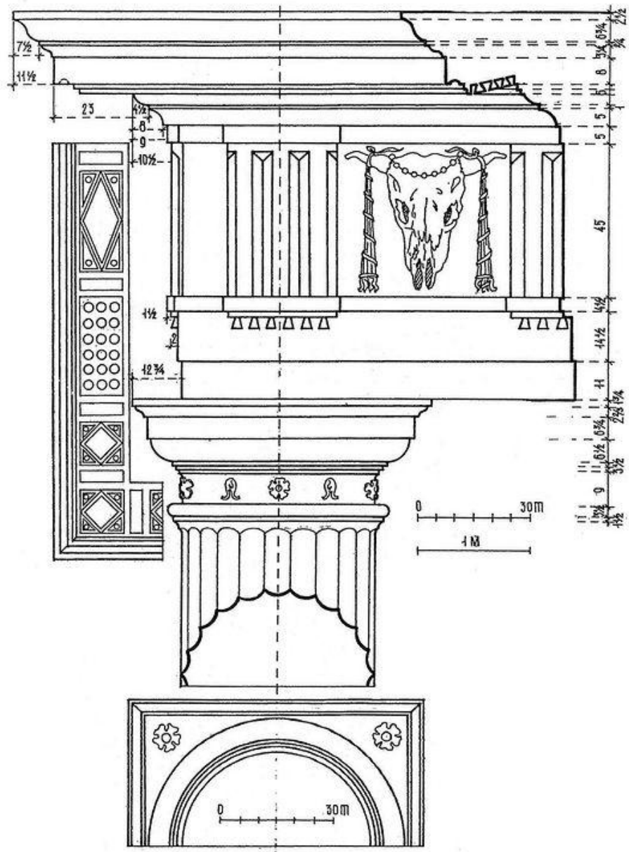
Палладио. Дорический ордер
