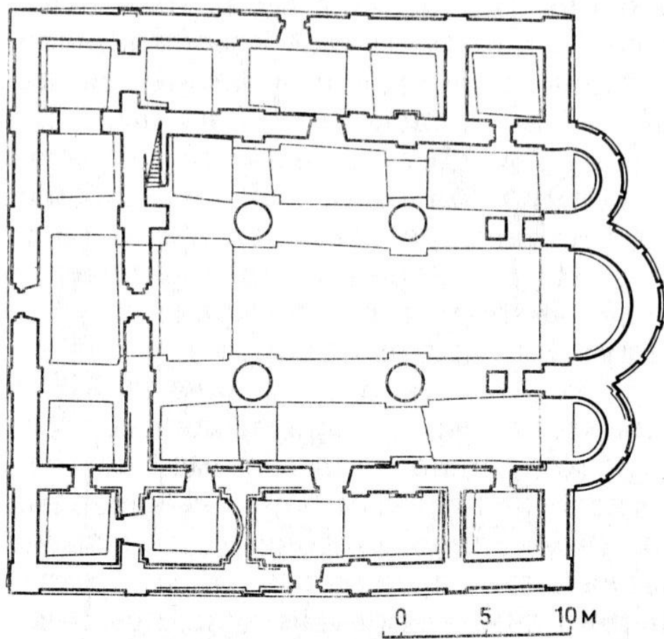
Галич. Успенский собор. Около 1157 г. План. Реконструкция Е. В. Воробьевой и А. А. Тица
