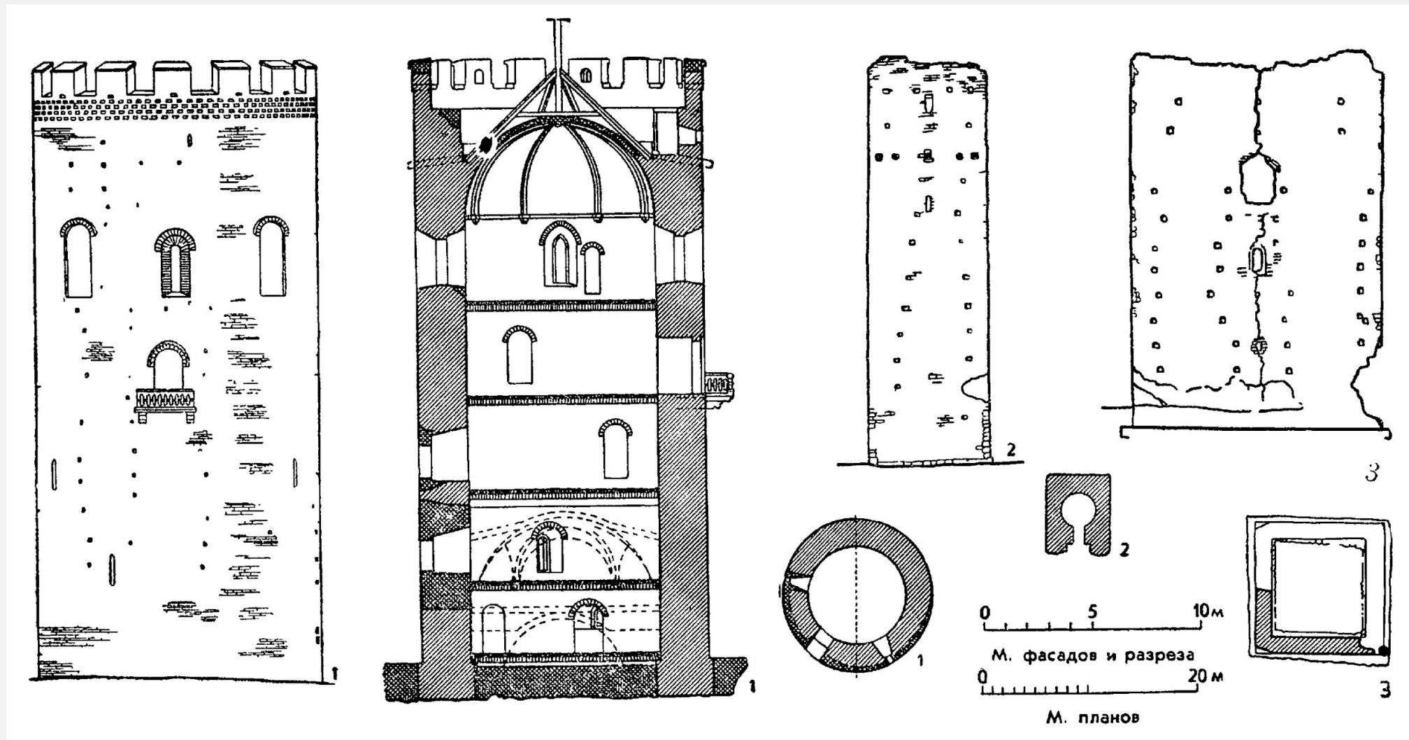
1 - Каменец-Литовский. Белая вежа, конец XIII в. (фасад, разрез и план); 2 - с. Столпье близ г. Холма. Башня, конец XIII в. (фасад и план); 3 - с. Белавино близ г. Холма. Башня, конец XIII в. (фасад и план)
