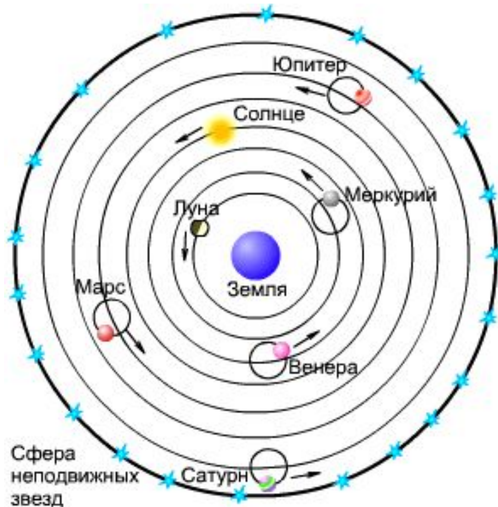
Геоцентрическая система Птолемея
