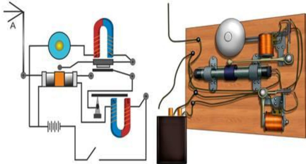
Схема приемника
