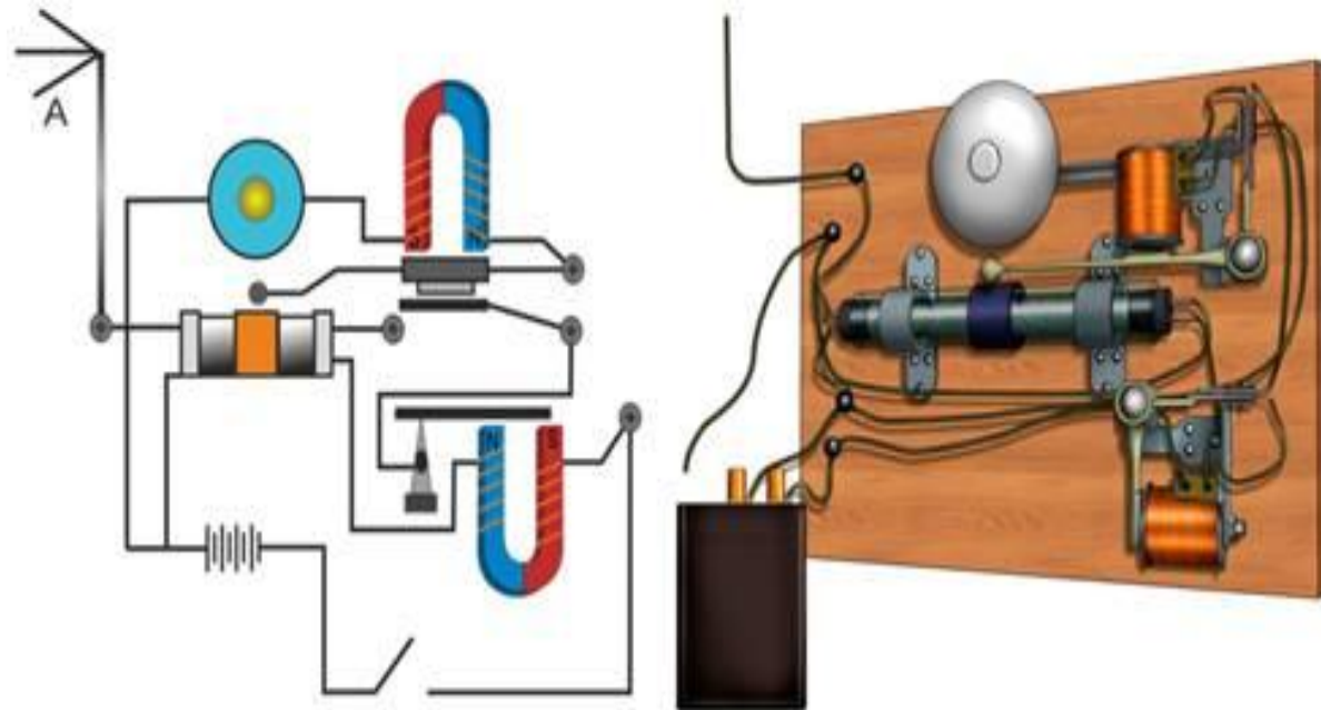
Схема приемника
