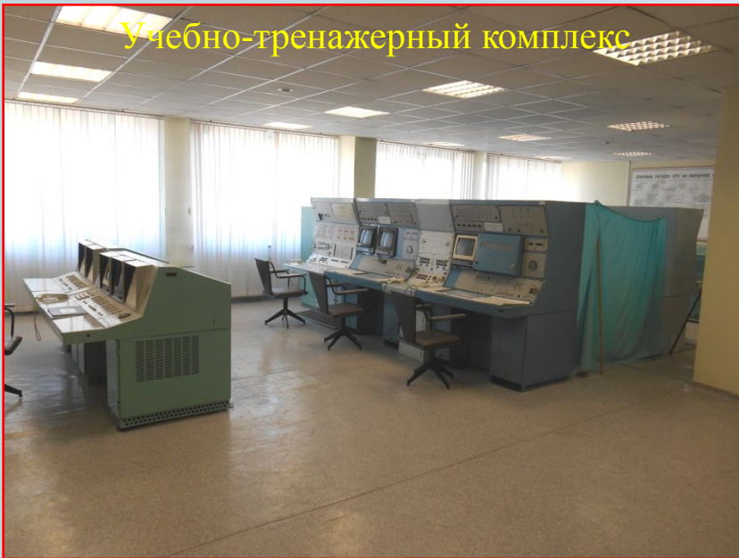
Учебно-тренажерный комплекс
