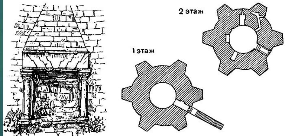
18. Конисборо. Цилиндрический донжон замка, 1185—1190 гг.
