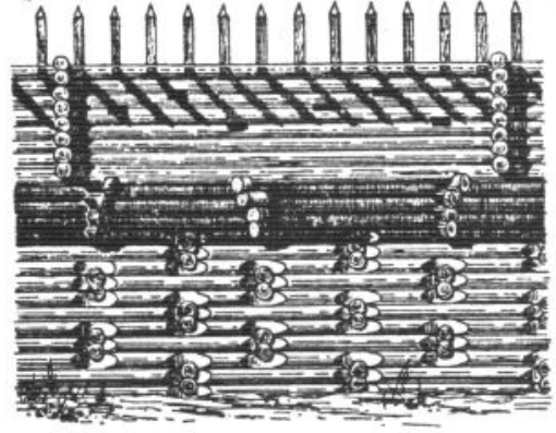
Фасадъ.
