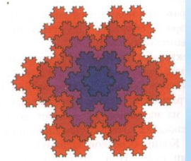
Рис. 5. Снежинка Коха
