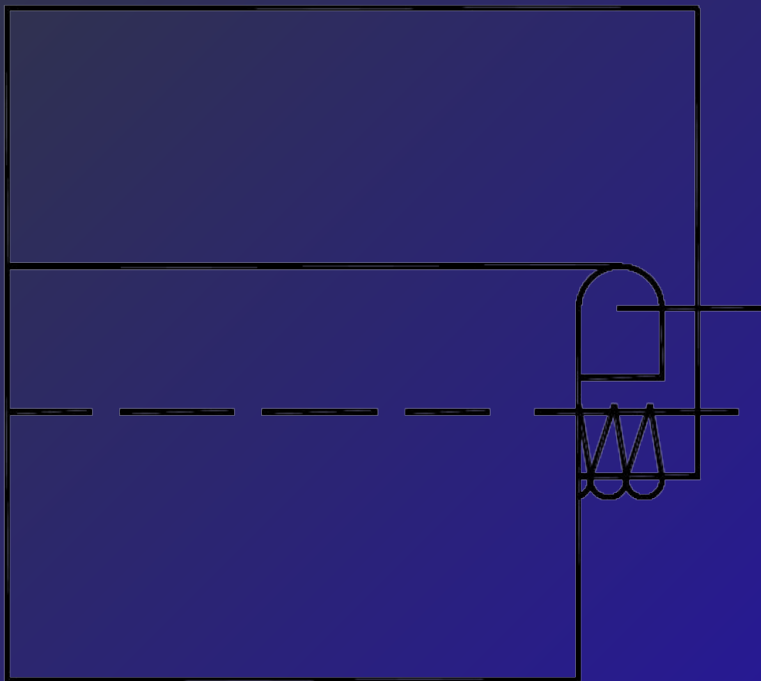
Рисунок 3. Схема соединения лифа с юбкой настрочным швом с закрытым срезом
