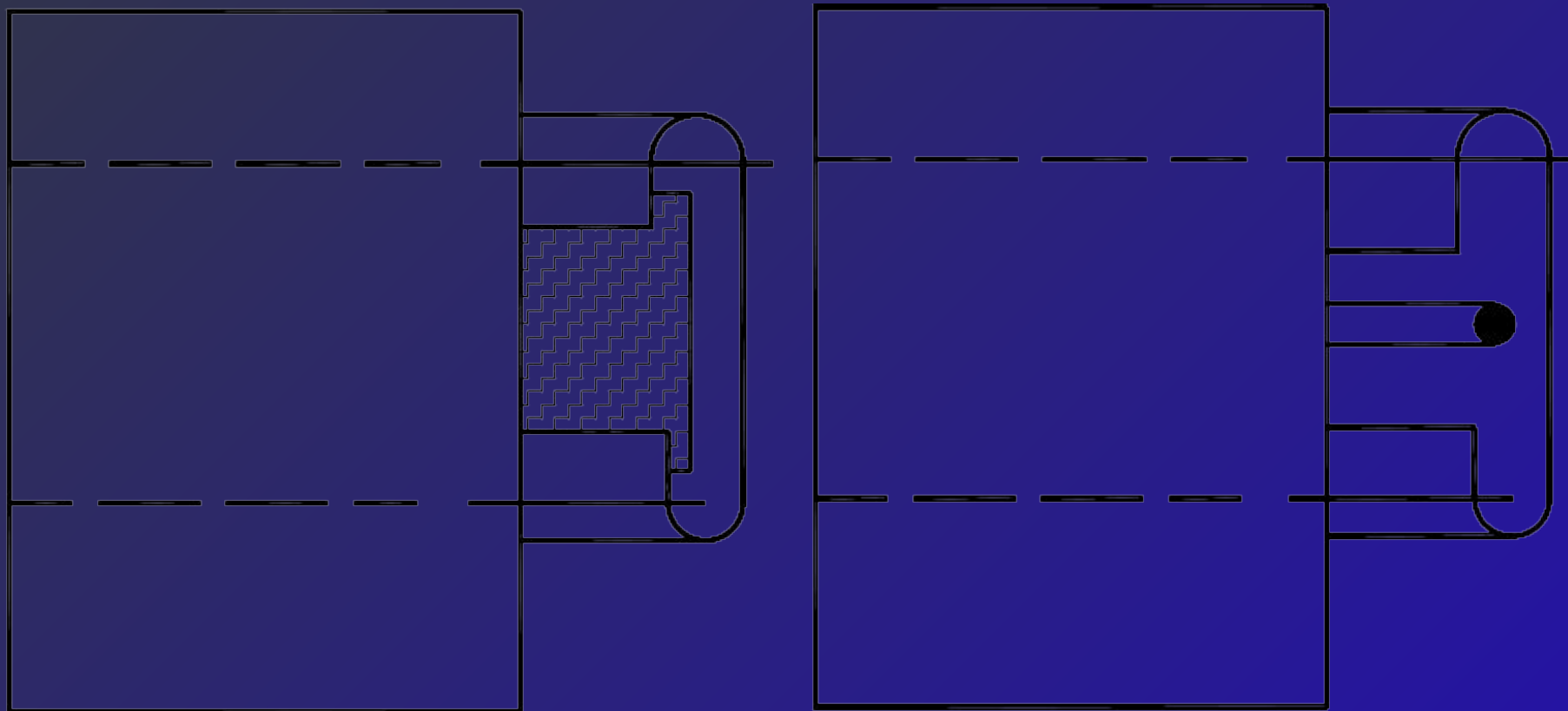
Рисунок 5. Схема соединения цельновыкроенного стана с «кулисой»
