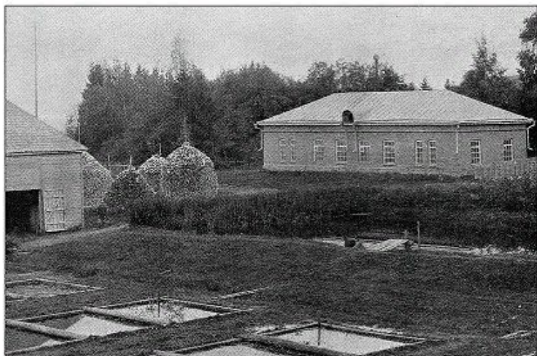
Машинное отделение Псковской опытной станции. Начало XX в.
