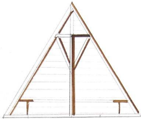
Вид А
