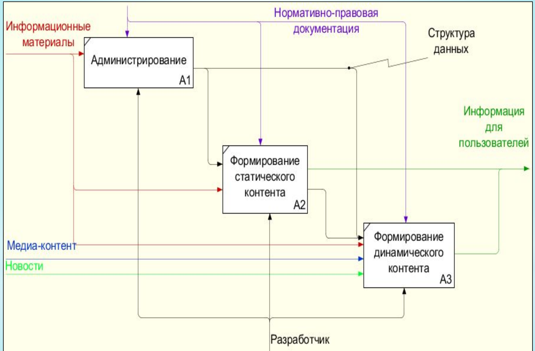
РИС. 2. ДЕКОМПОЗИЦИЯ ДИАГРАММЫ
