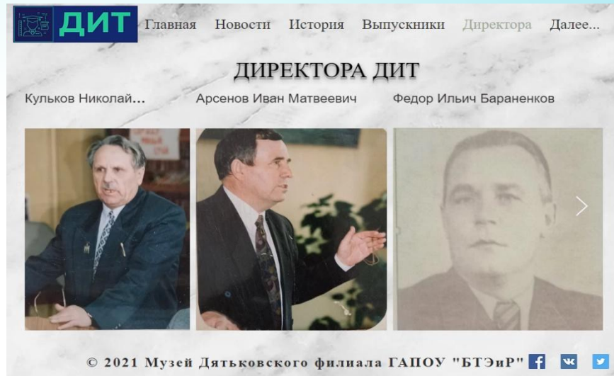
РИС.5. РАЗДЕЛ «ДИРЕКТОРА»
