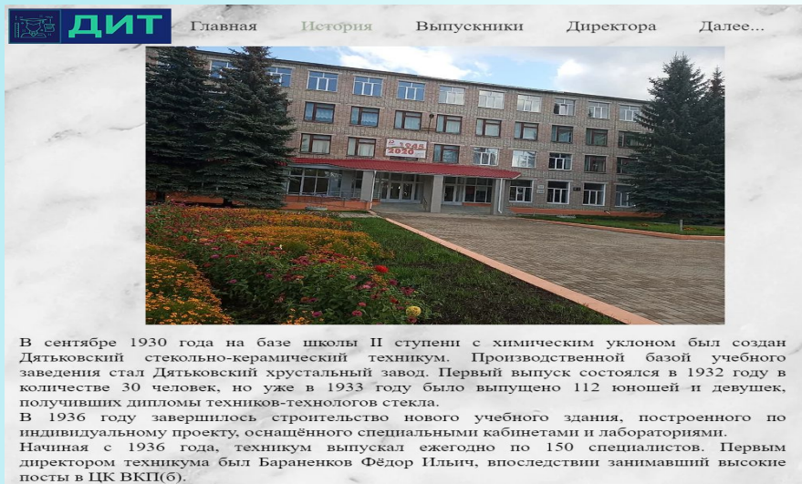
РИС.4. РАЗДЕЛ «ИСТОРИЯ»
