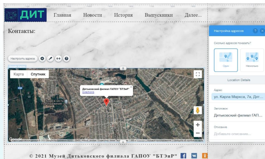
РИС.10. РАЗДЕЛ «КОНТАКТЫ»
