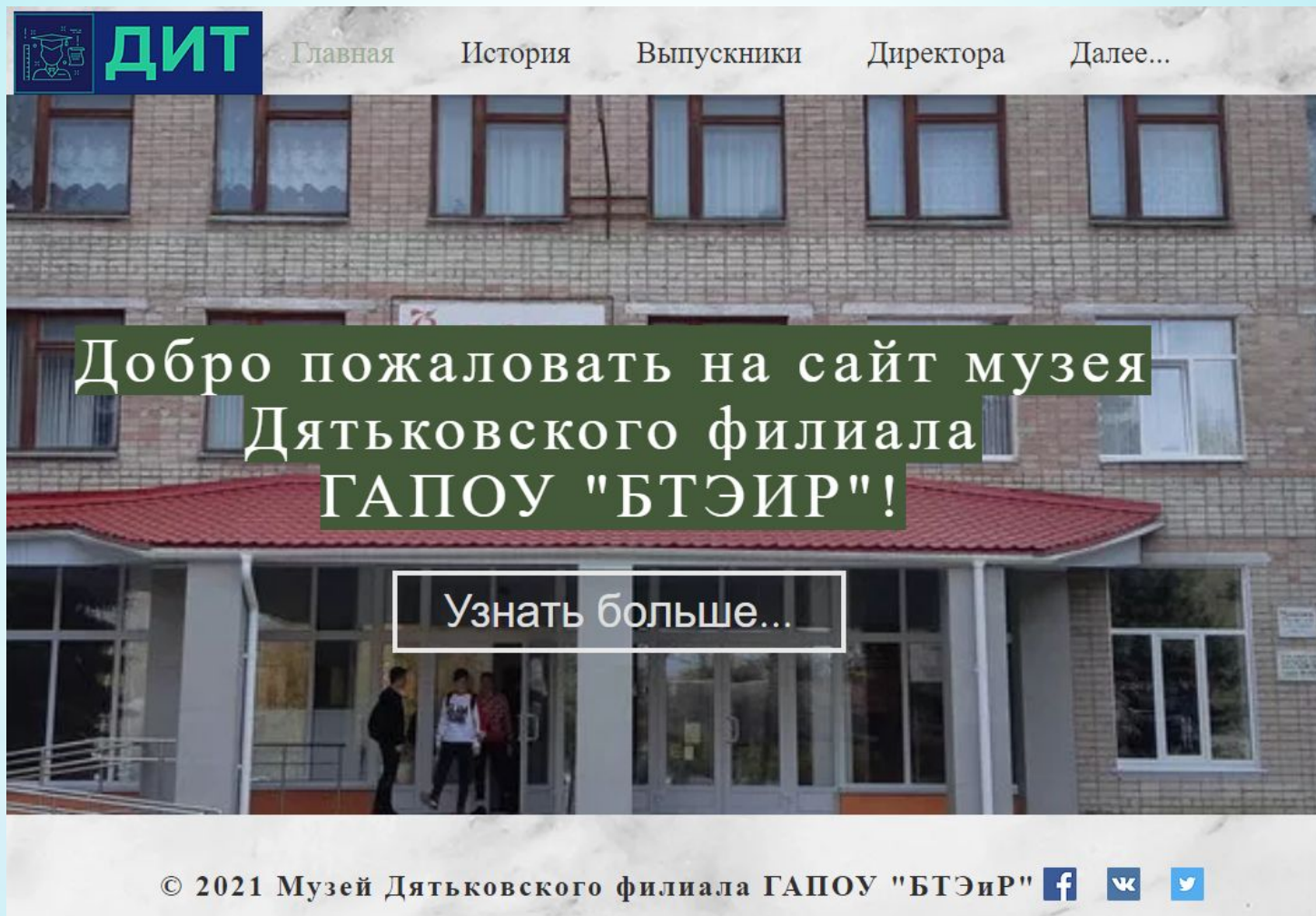
РИС. 3. ГЛАВНАЯ СТРАНИЦА
