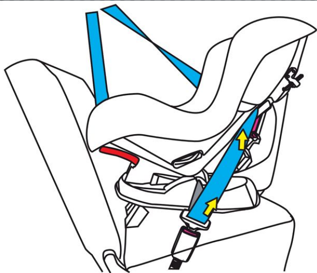
Установка ремennого кресла спиной вперед
