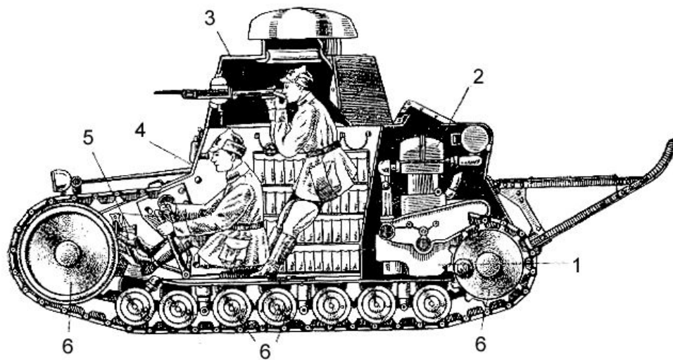
Рис. 2. Продольный разрез танка.
