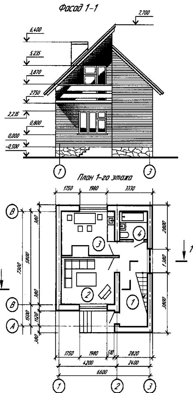
Рис. 298. Фасад и план дома
