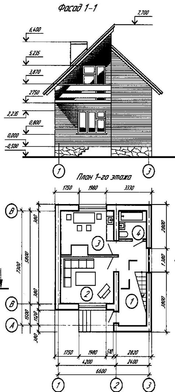
Рис. 298. Фасад и план дома
