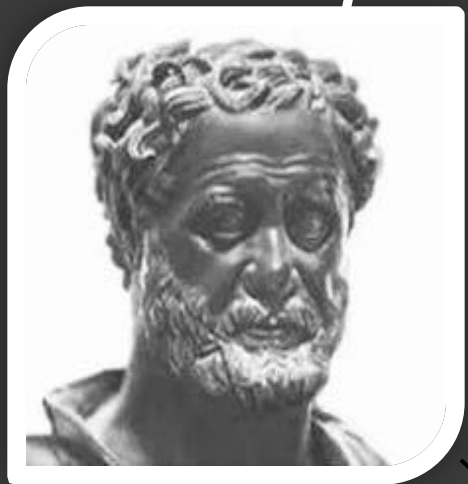
Линия Гераклита
