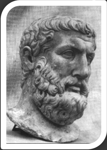
Линия Парменида
