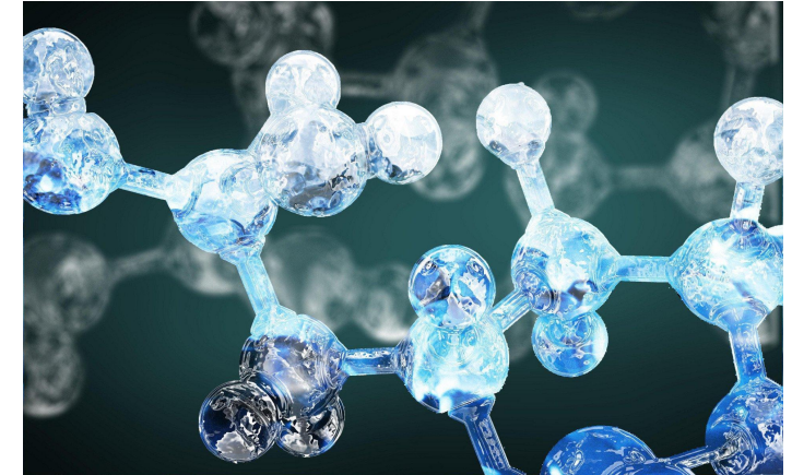
Отвердевшие молекулы
