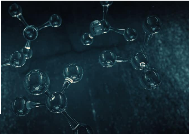
Молекулы клея
