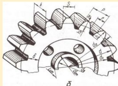
Рисунок 1 – Елементи зубчастого колеса
