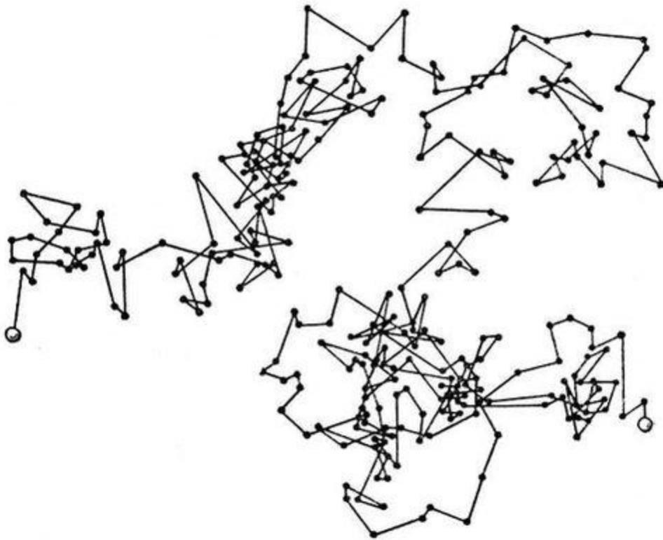
Броуновское движение
