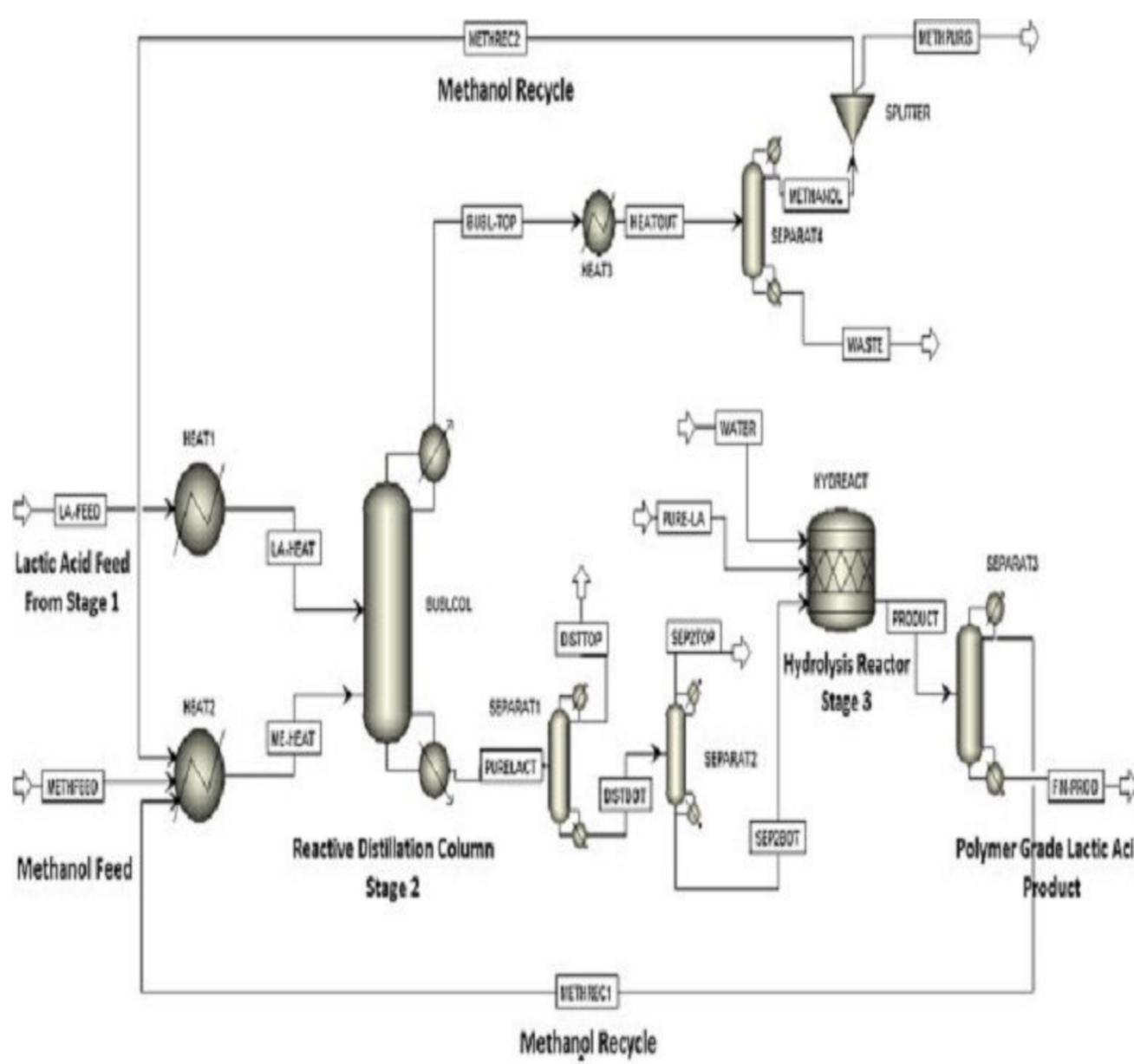
شکل 2 دیاکرام فرآیند تولید
