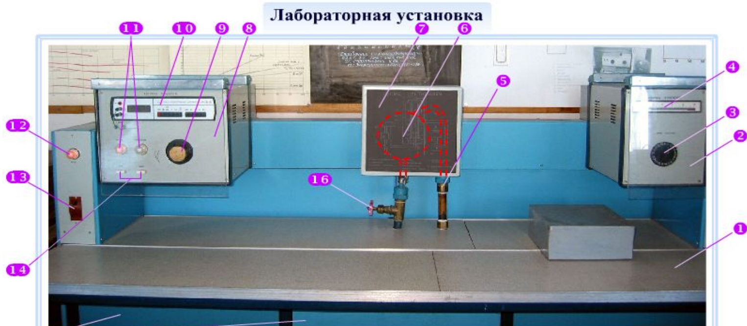
Рис. 1. Внешний вид лабораторной установки
