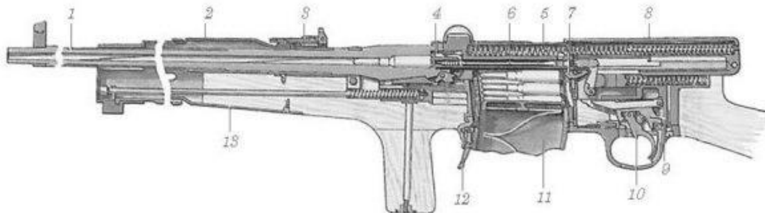
Положение частей и механизмов автомата в момент выстрела: 1 — ствол; 2 — ствольная накладка; 3 — прицел; 4 — патронник; 5 — ударник; 6 — возвратная пружина; 7 — курок; 8 — корпус; 9 — спусковой механизм; 10 — спусковой крючок; 11 — магазин; 12 — защелка магазина; 13 — ложа
