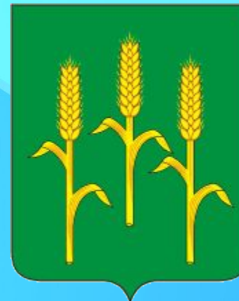
Мещовский
