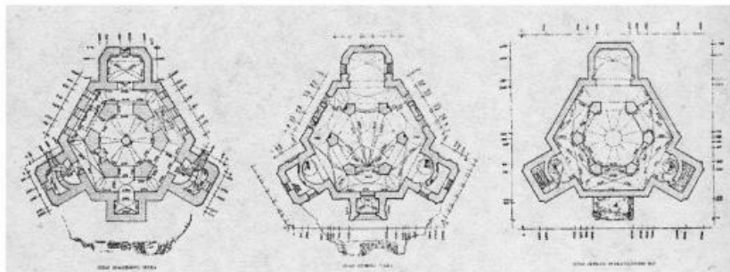
СТАРАЯ ОЛЬШАНКА Церковь Воскресения Христа Спасителя 1843-1860. Арх. Р.И.Кузьмин (фасады), худ. К.А.Молдавский (план) Обмерные чертежи И.Ю.Поздняковой
