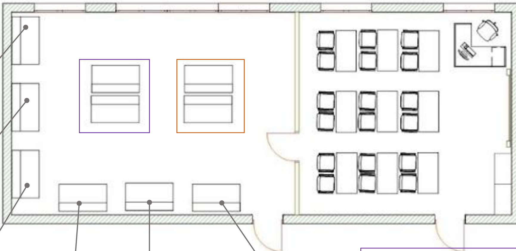
Типовой комплект учебного оборудования «Гидравлические сопротивления водопроводной арматуры»
