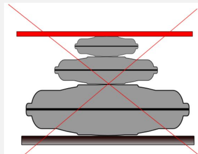
Rysunek nr 13. Niepoprawne zastosowanie siłowników [1,2,3].
